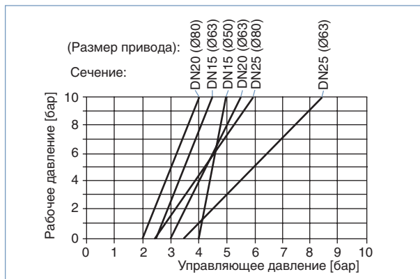
Диаграмма 3 – сечение 15-25
