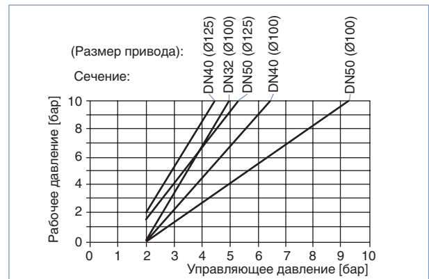
Диаграмма 2 – сечение 32-50
