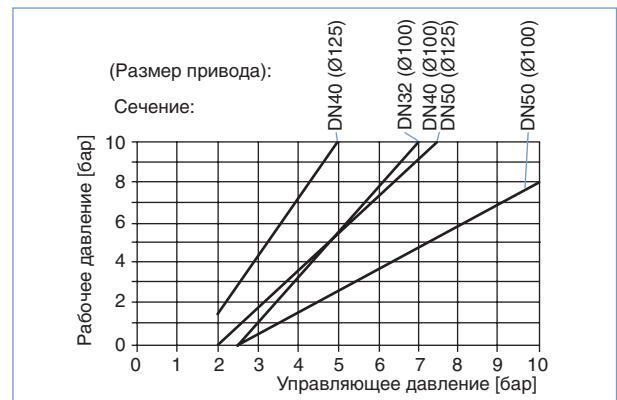
Диаграмма 4 – сечение 32-50
