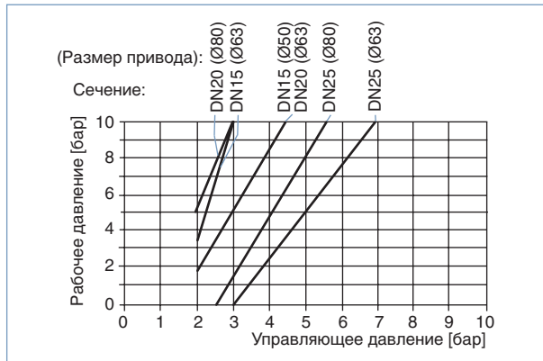
Диаграмма 1 – сечение 15-25
